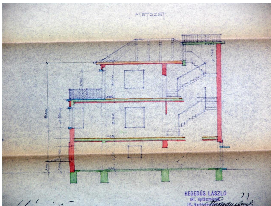
13. kép Metszet
