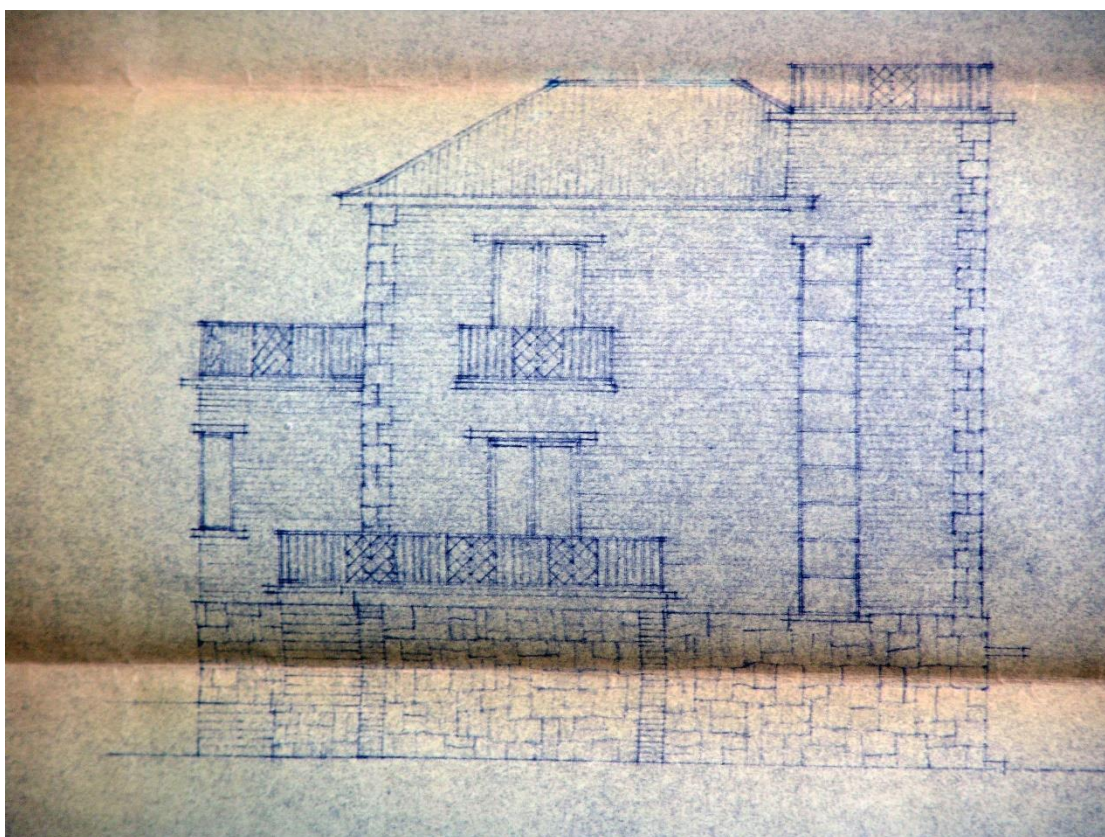
11. kép Oldalhomlokzat
