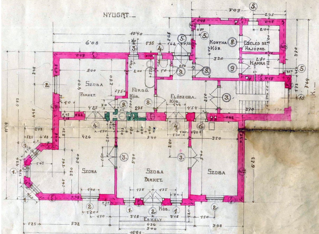
4. kép Földszinti alaprajz, 1910
