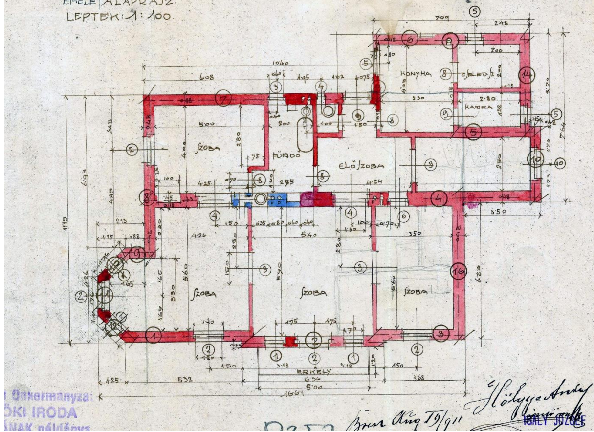
5. kép Emeleti alaprajz
