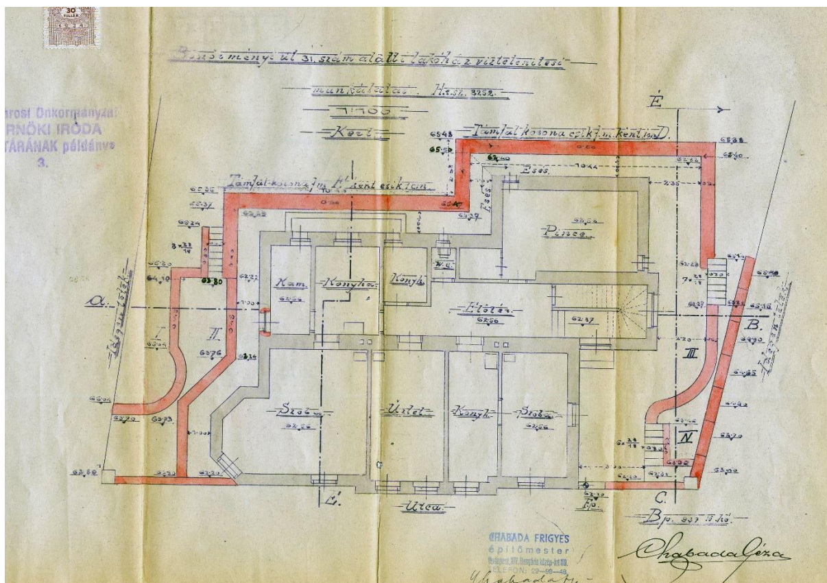
15. kép Vízvezetés terve, 1937
