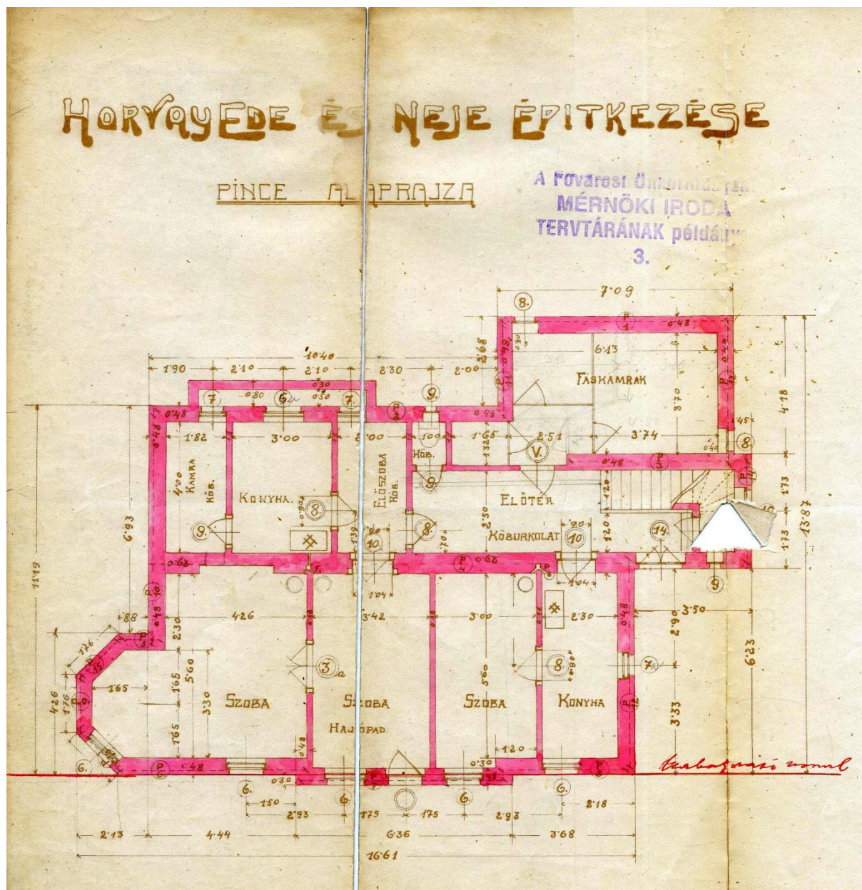
3. kép Kivitelezési terv, pince
