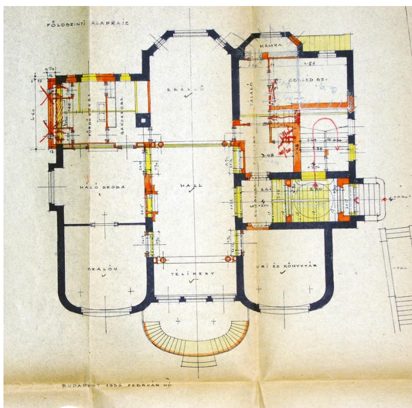
3. kép Földszint alaprajz, tervvariáns, 1936
