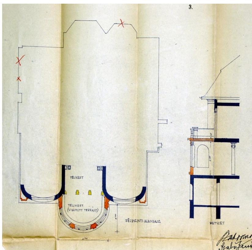
5. kép Földszint, alaprajz és metszet, tervvariáns, 1936
