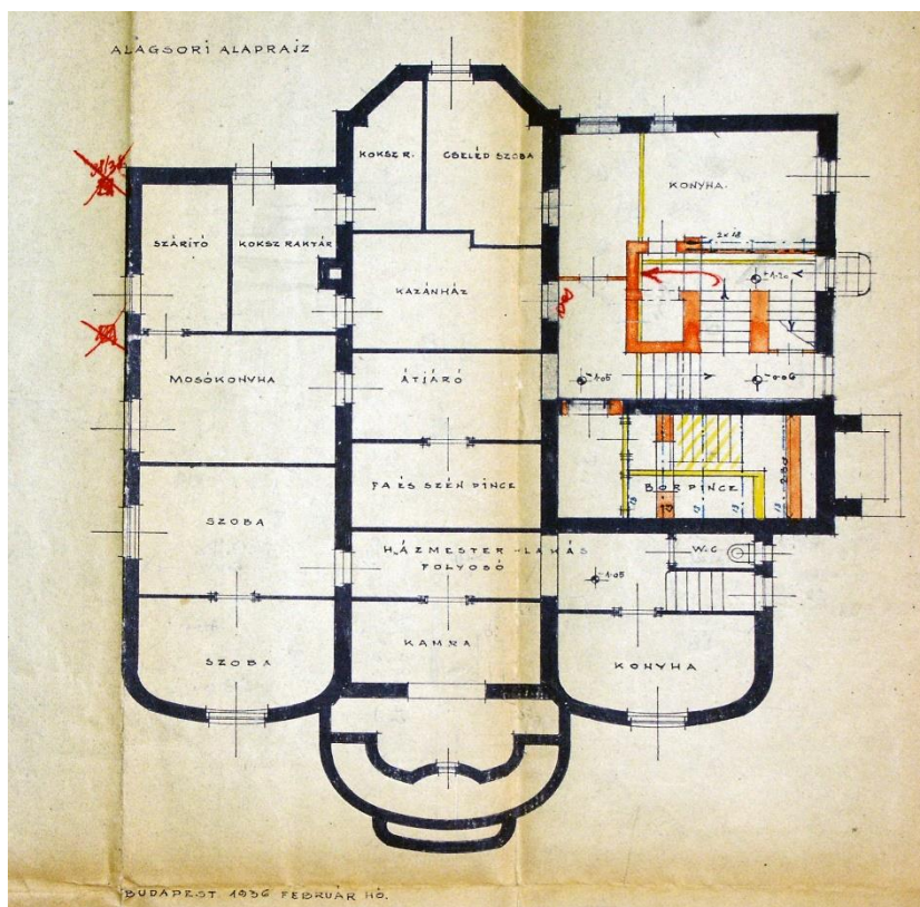
2. kép Alagsor, alaprajz, tervvariáns, 1936
