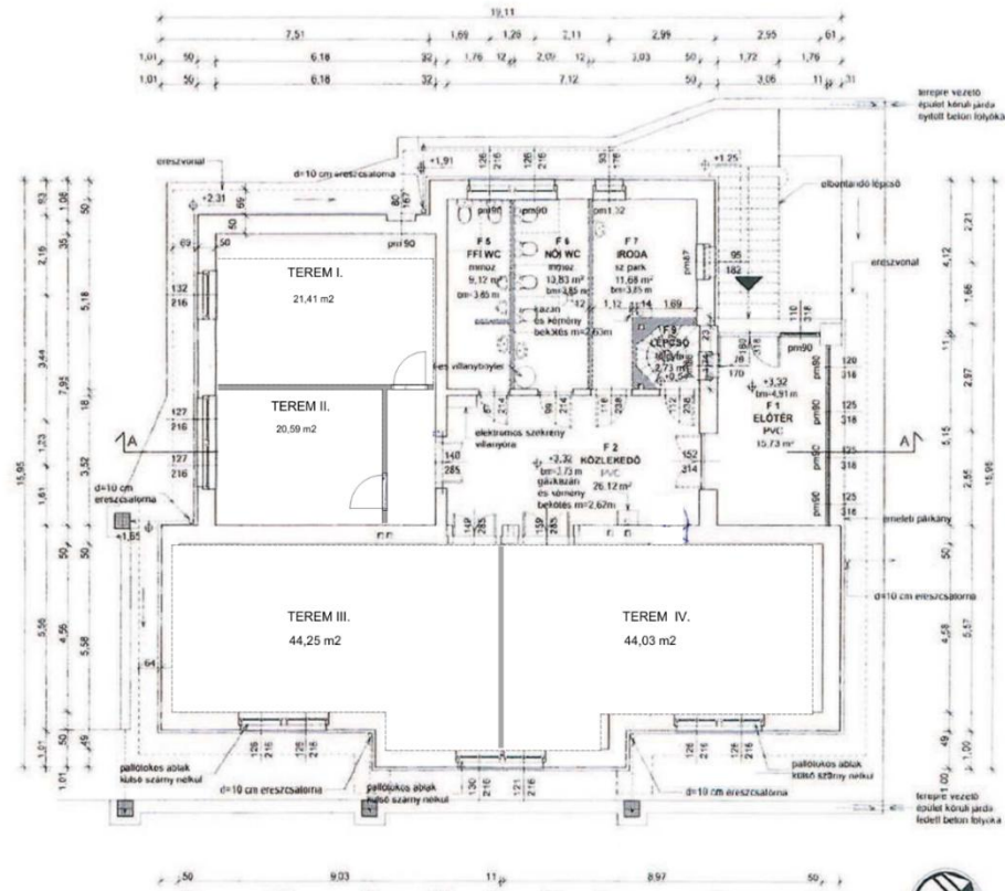
Alaprajz
