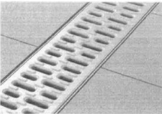
Folyóka típusa ACO V100G (13,5x15 cm), horganyzott acél ráccs:
